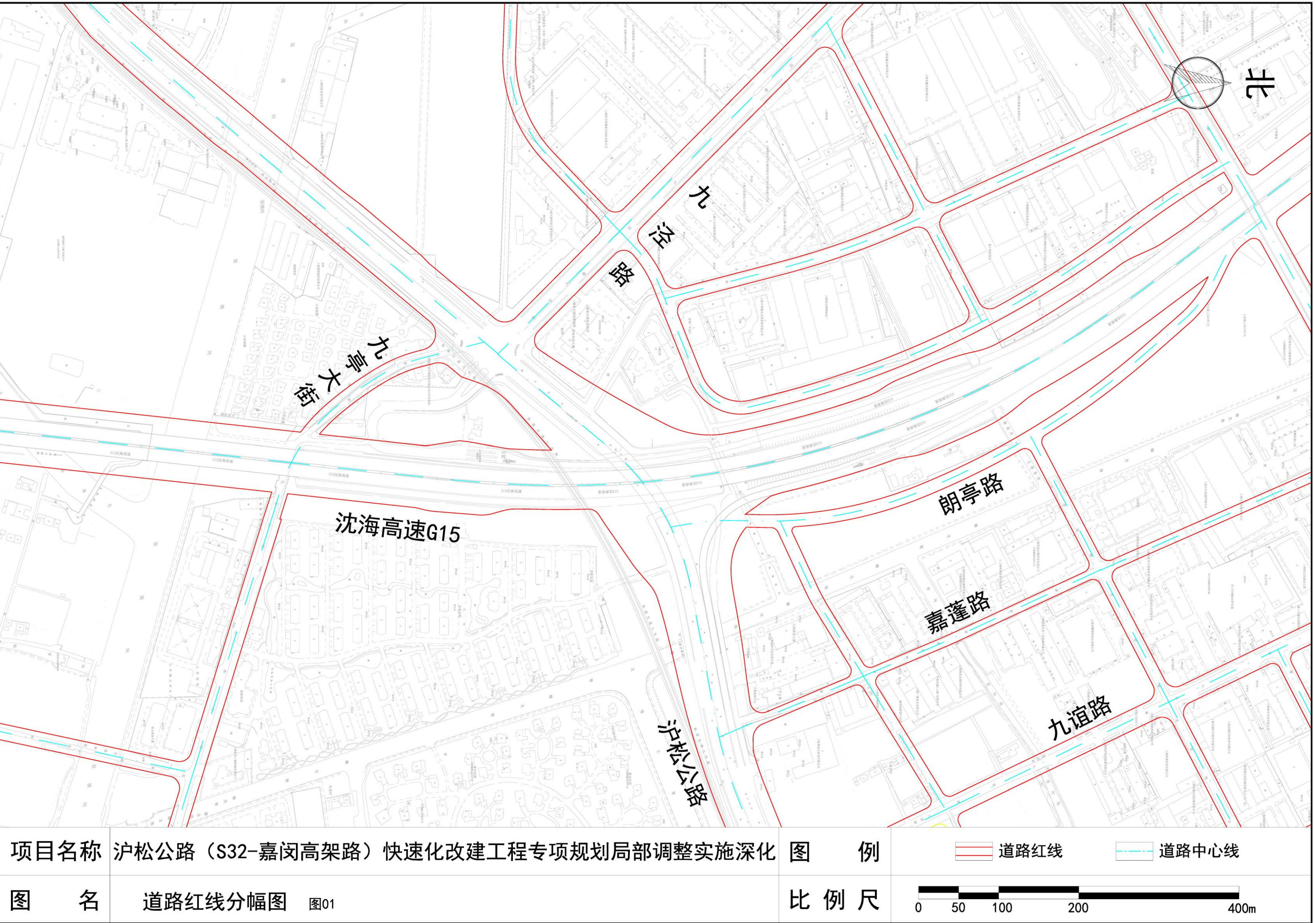
道路红线分幅图（1/4）
